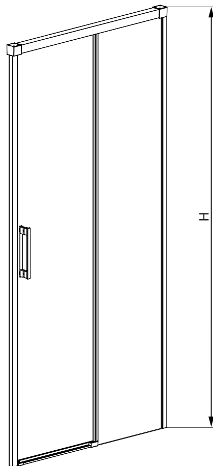
Pravostranné dvere Variant R
